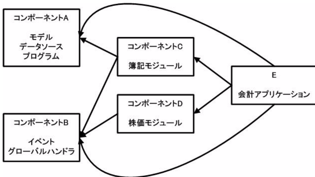
図 7-1 ネストされたコンポーネントシステムの例
